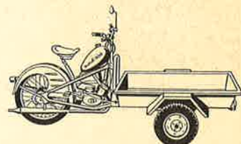
Mokuli 250 A (Grundtype)
