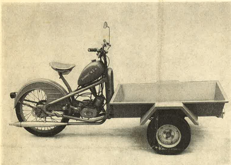
Mokuli 250 A (Grundtype)
